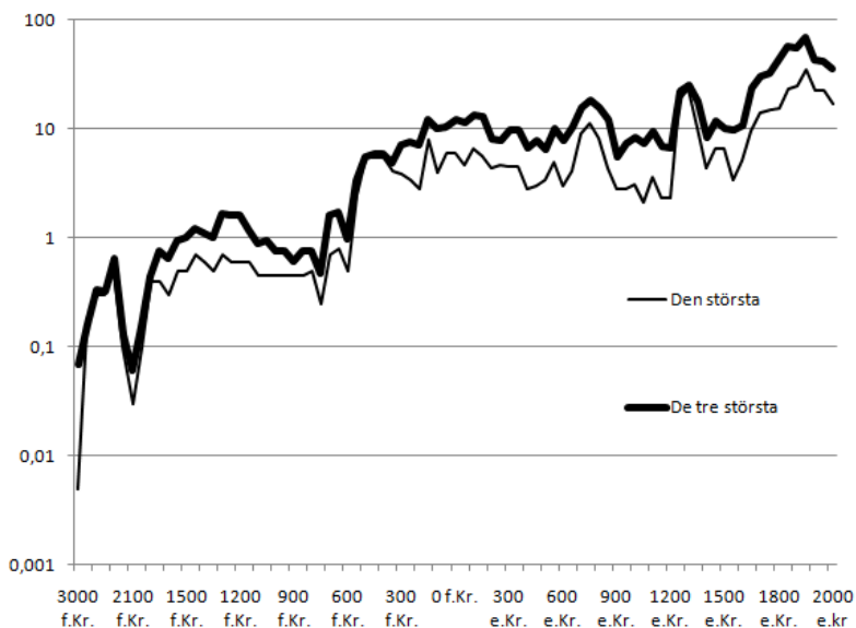
FIGUR 1. Taageperas kurva över den största och de tre största staterna. Kurvan är semi-logaritmisk, så att även förändringen under den tidigaste perioden framgår. Kurvan har korrigerats efter de skilda uppgifter som Taagepera anger i olika artiklar. Dessutom har utvecklingen fram till år 2000 medtagits.
